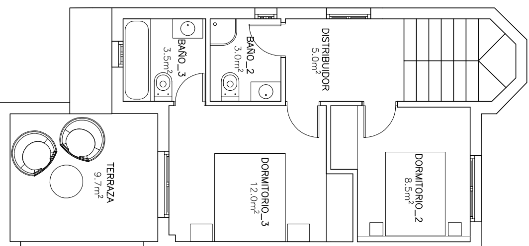
PLANTA PRIMERA
