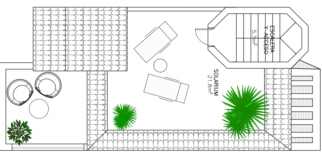
PLANTA SOLARIUM
